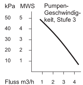
Druckverlustdiagramm
